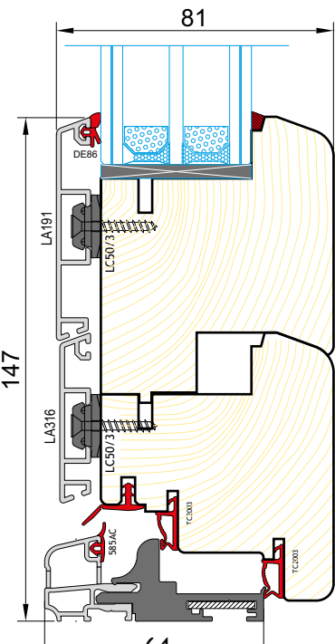
Porta parte bassa Lower section door
