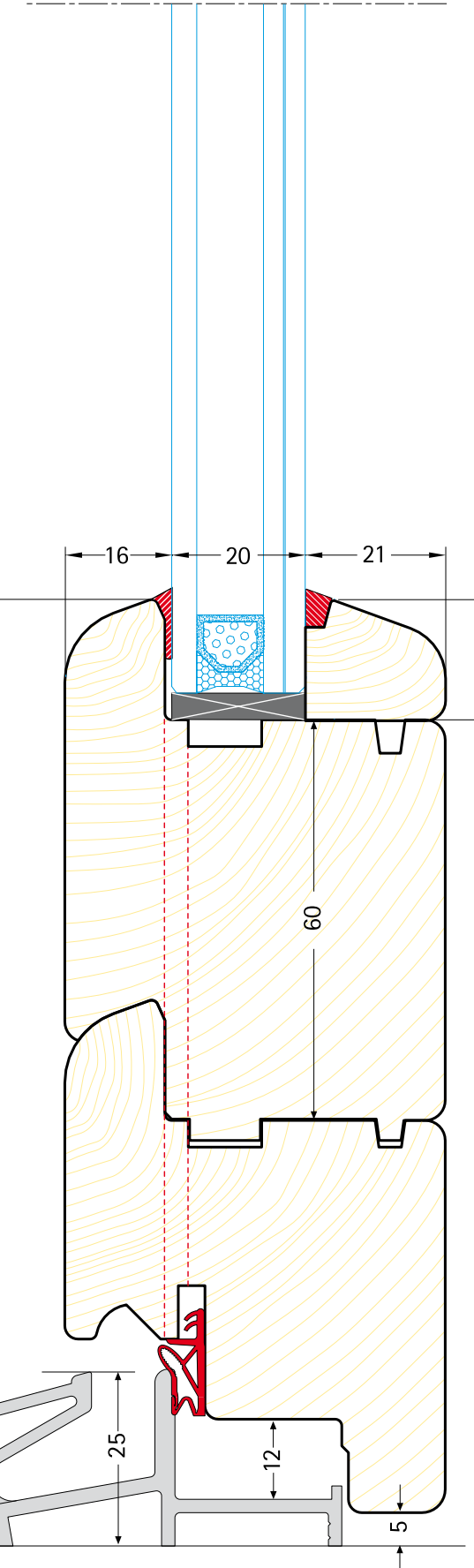
Portafinestra parte bassa Lower section door
