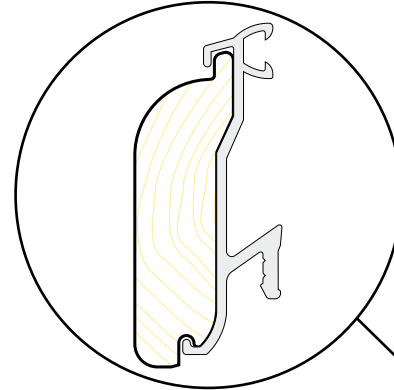
Variante gocciolatoio rivestito legno Wood clad drip
